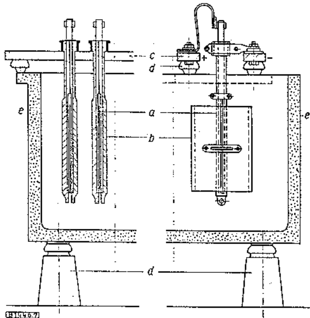
Abb. 7. Elektrolyse-Zellen beim Chedde-Verfahren. a Anode, b Kathode, c Stromzuführungen, d Porzellan-Isolierung, e Beton-Trog
